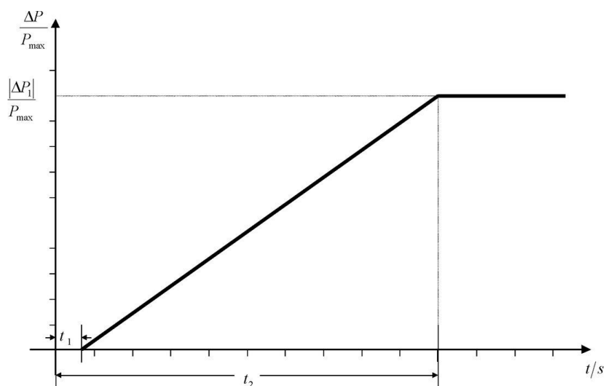
Slika 6.17: Sposobnost frekvencijskog odziva djelatne snage HVDC sustava.
