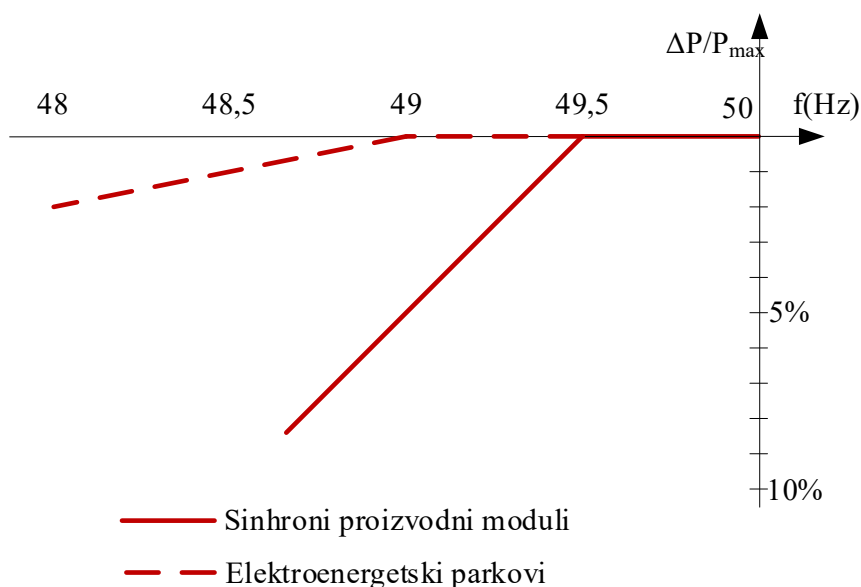
Slika 6.3. Najveće smanjenje izlazne snage s opadanjem frekvence
