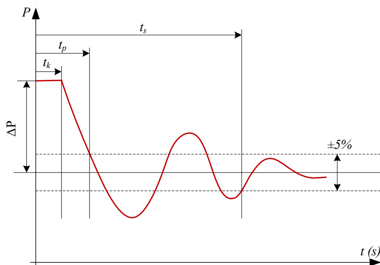
Slika 6.1. Tolerancija i trajanje odziva djelatne snage
