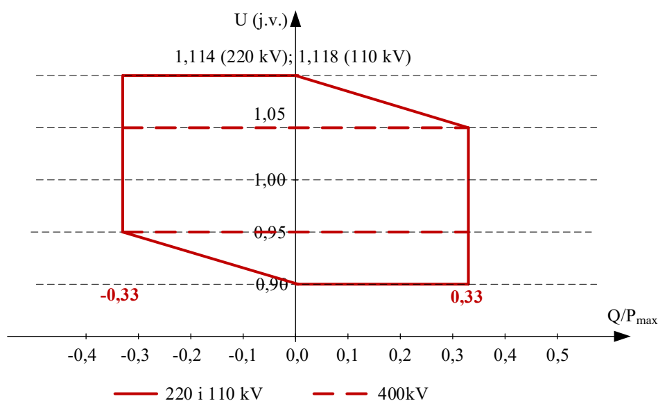
Slika 6.20. Karakteristika U-Q/P_{\max} HVDC sustava na mjestu priključenja na prijenosnu mrežu
