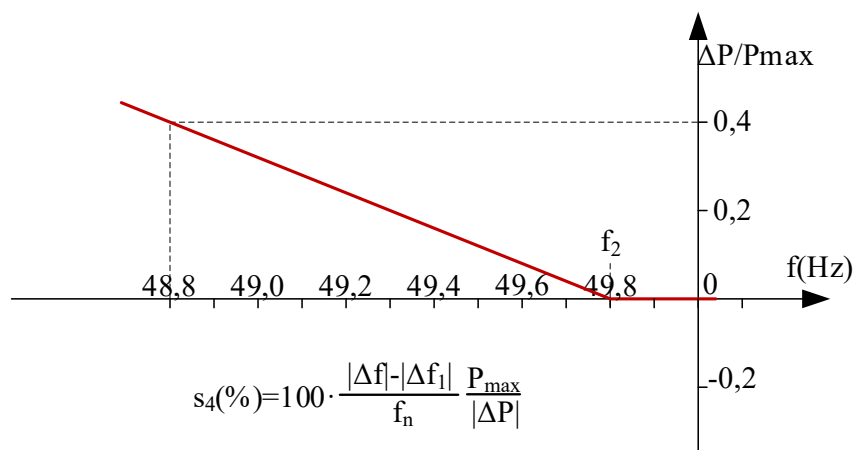
Slika 6.19: Spособnost HVDC sustava za frekvencijski odziv djelatne snage u LFSM-U-u.
