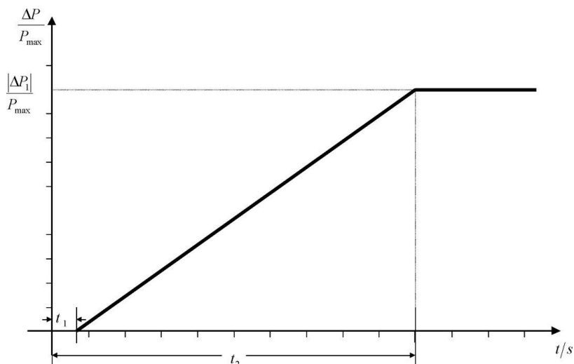
Slika 6.9. frekvencijski odziv djelatne snage
