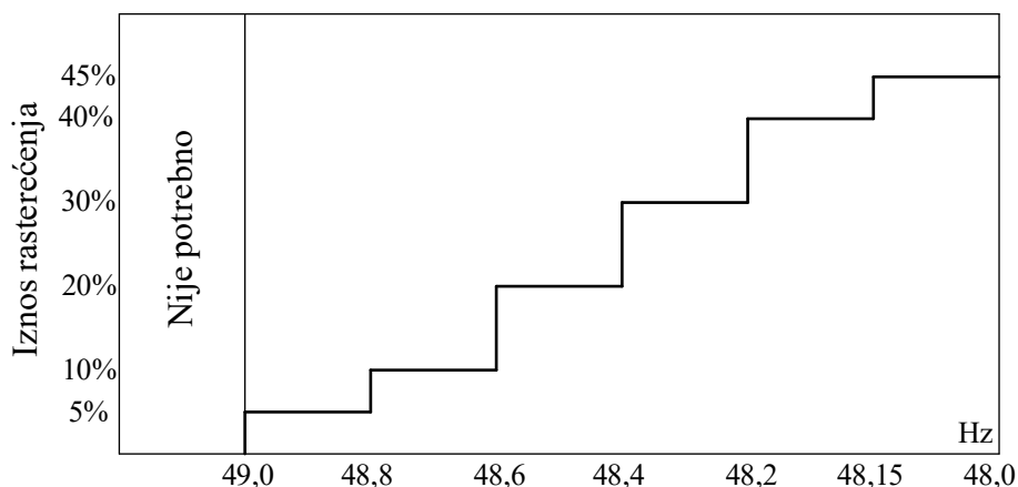
Slika 8.1. Opsezi podešenja releja podfrekvencijske zaštite
