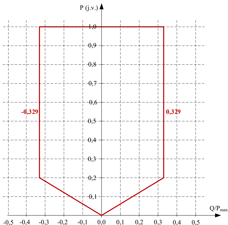
Slika 6.21. Karakteristika P-Q/P max HVDC sustava na mjestu priključenja na prijenosnu mrežu
