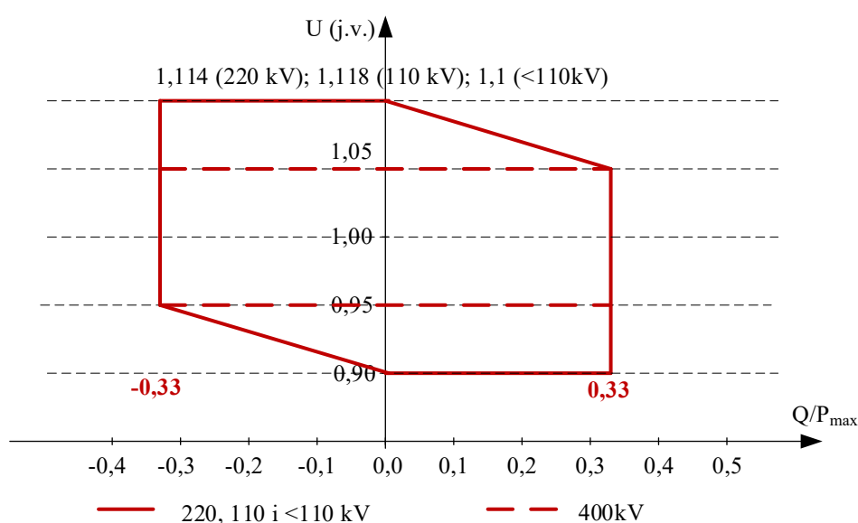
Slika 6.11. Karakteristika U-Q/P_{\max} modula elektroenergetskog parka
