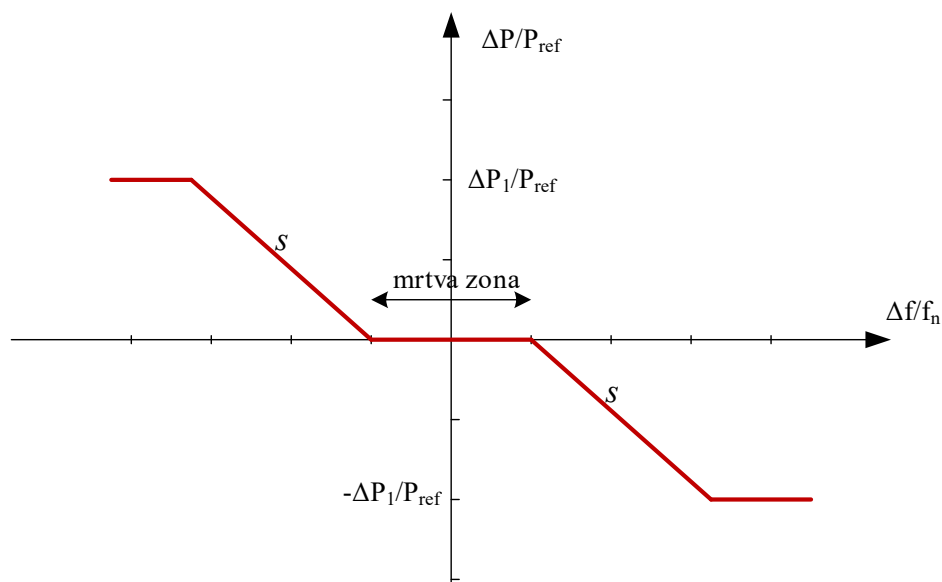
Slika 6.8. Frekvencijski odziv djelatne snage u frekvencijsko osjetljivom načinu rada
