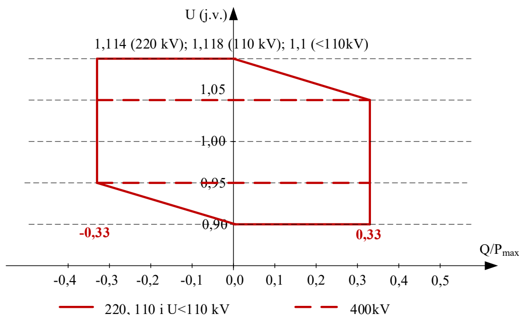
Slika 6.10. Karakteristika U-Q/P_{\max} sinkronog proizvodnog modula
