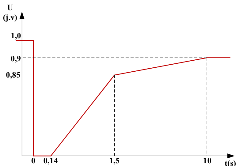
Slika 6.22. FRT za HVDC sustave u točki priključenja na prijenosnu mrežu
