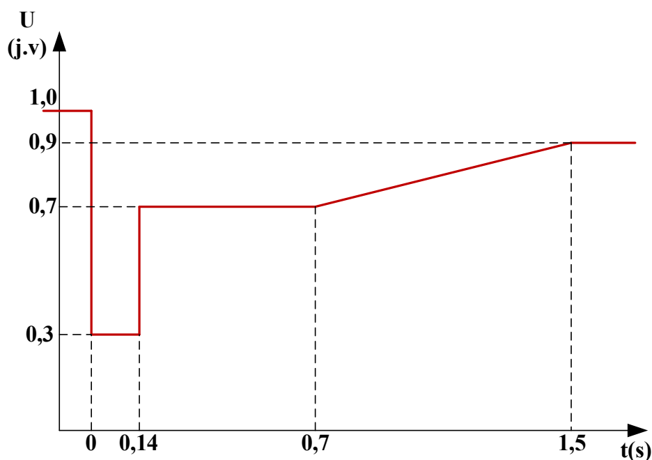
Slika 6.4. FRT kriva za sinkrone proizvodne module
