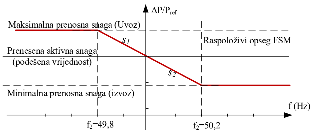
Slika 6.16: Frekvencijski odziv djelatne snage HVDC sustava
