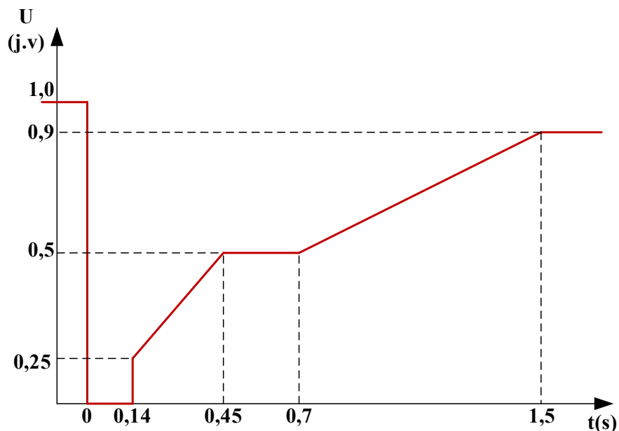
Slika 6.13. FRT kriva za sinkrone generatore
