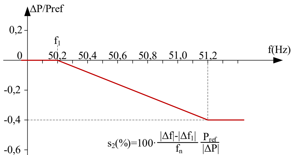
Slika 6.2. Frekvencijski odziv djelatne snage u LFSM-O
