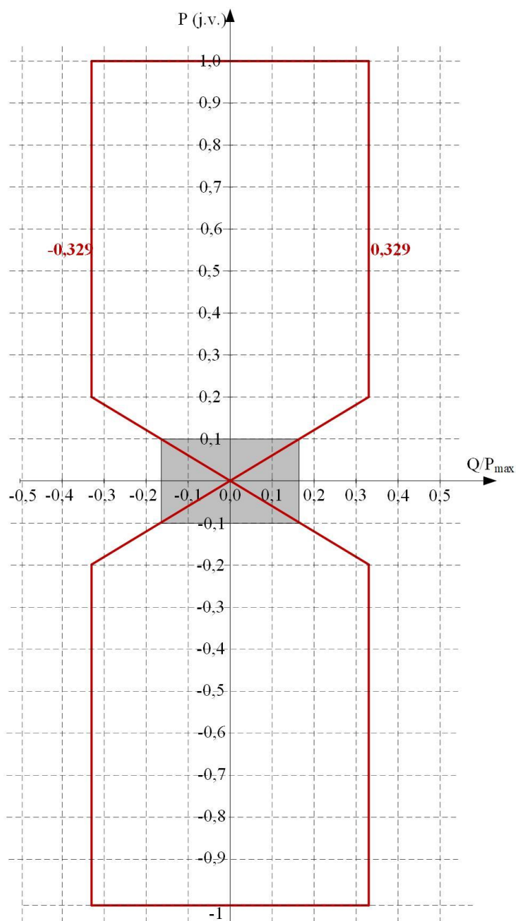
Slika 6.24. Pogonska karta za jalovu snagu
