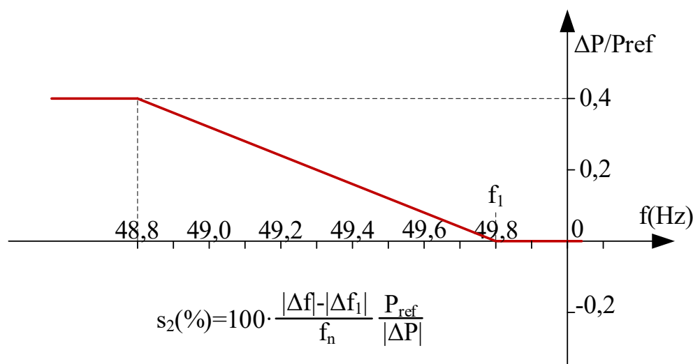
Slika 6.7. Frekvencijski odziv djelatne snage u LFSM-U
