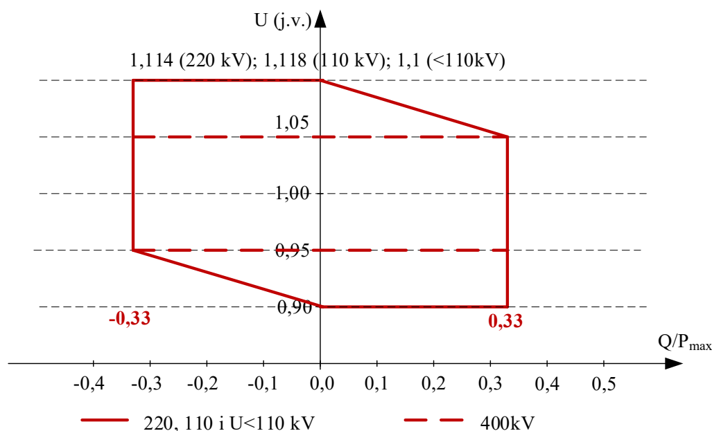
Slika 6.10. Karakteristika U-Q/P_{\max} sinhronog proizvodnog modula
