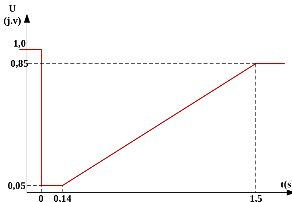
Слика 6.5. FRT крива за модуле електроенергетских паркова
